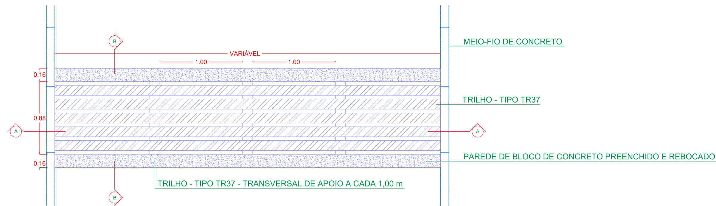
DETALHE - PLANTA BAIXA - TRINCHEIRA ESC. 1:50
