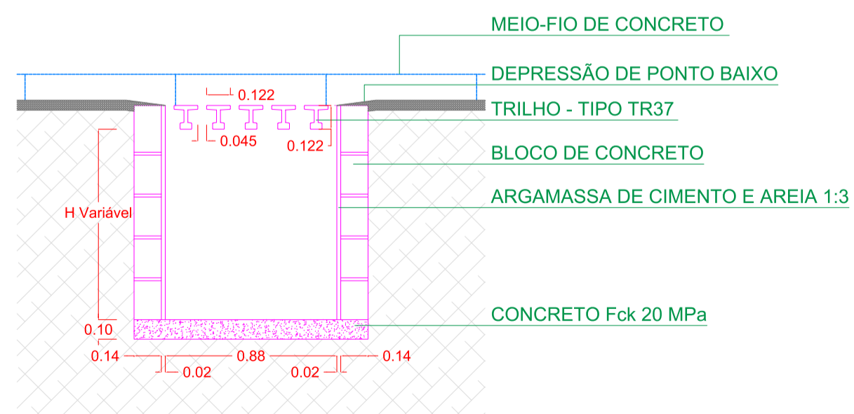
DETALHE - CORTE A-A ESC. 1:50
