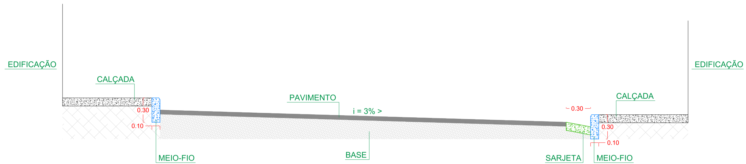
DETALHE - CORTE - RUA ESC. 1:50
