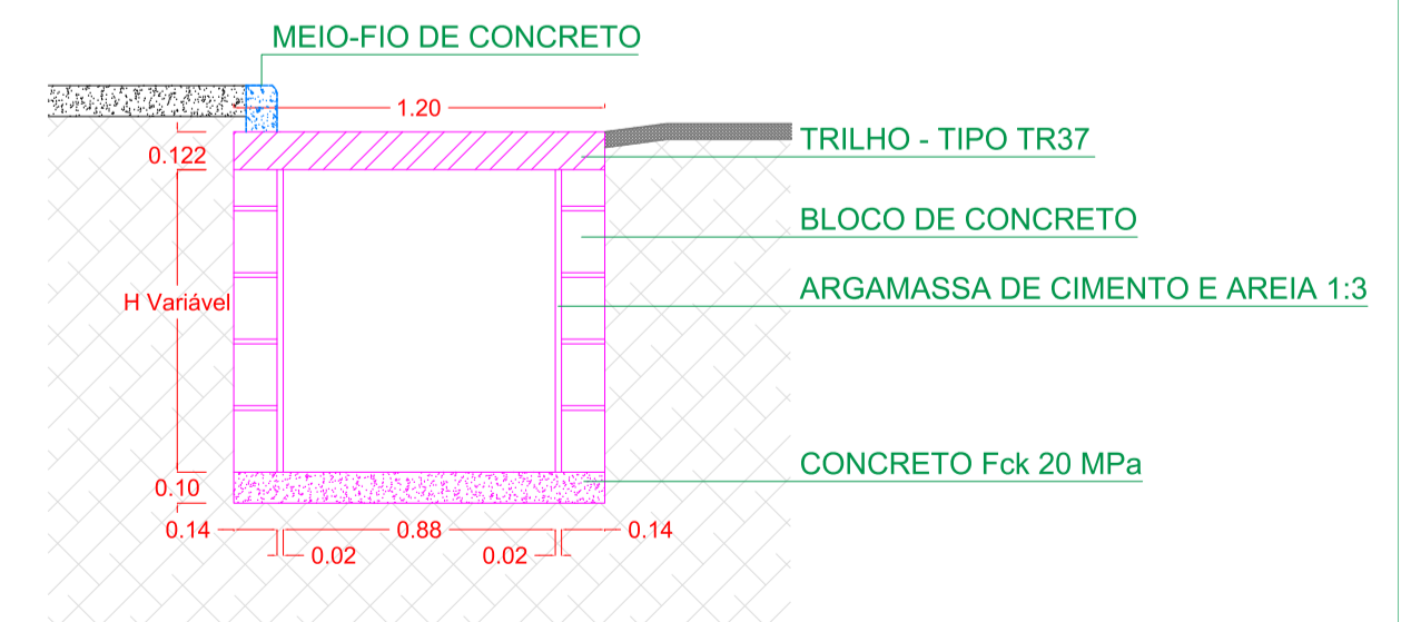
DETALHE - CORTE B-B ESC. 1:50
