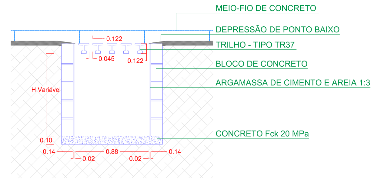
DETALHE - CORTE B-B ESC. 1:50
