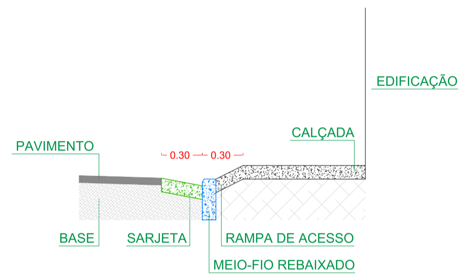
DETALHE - CORTE - ENTRADA DE GARAGEM ESC. 1:50
