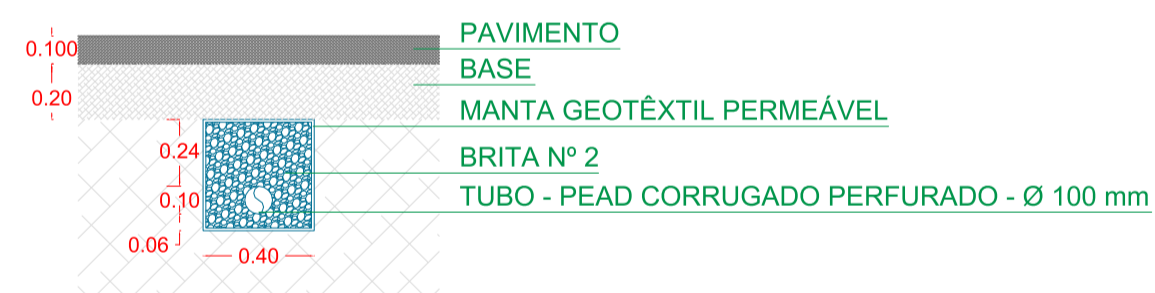
DETALHE - DRENO SUBSUPERFICIAL ESC. 1:50
