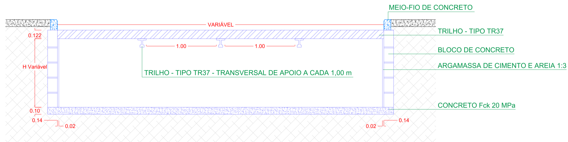
DETALHE - CORTE A-A ESC. 1:50
