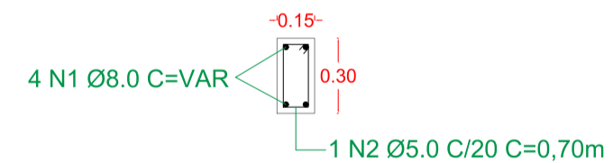
DETALHE - VIGA DE TRAVAMENTO - BLOQUETAMENTO ESC. 1:50
