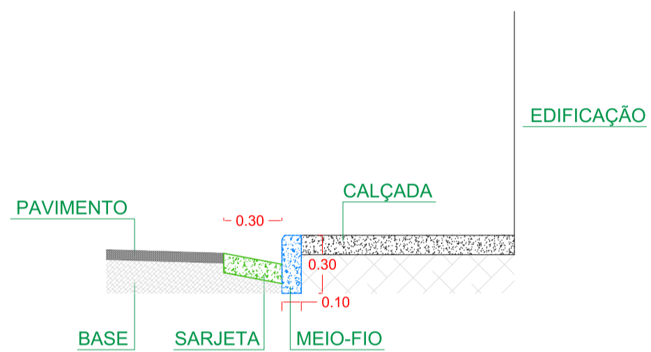
DETALHE - CORTE - SARJETA E MEIO-FIO ESC. 1:50
