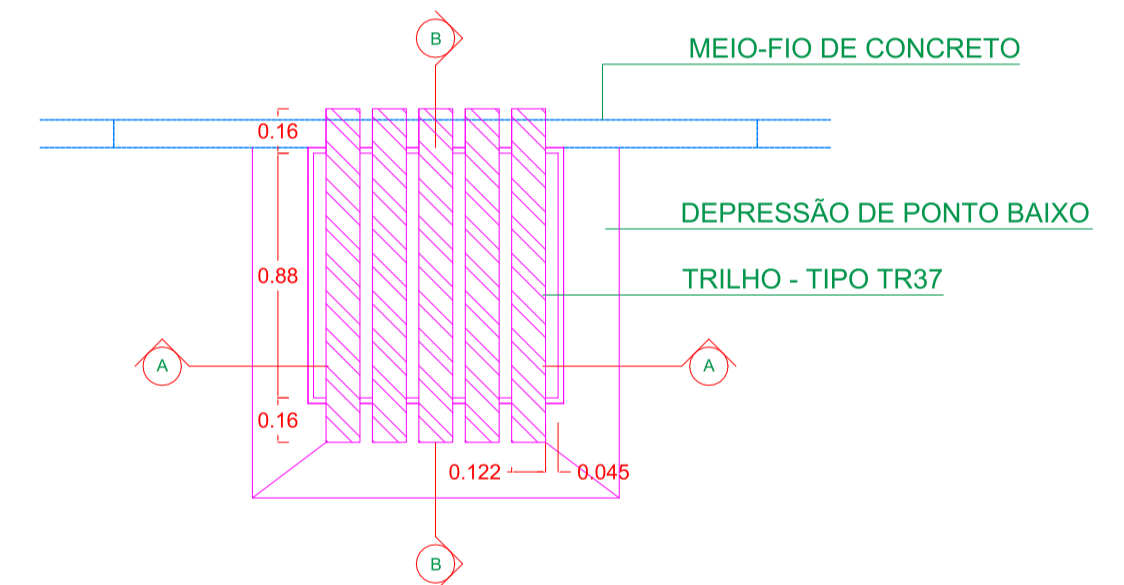
DETALHE - PLANTA BAIXA - BOCA-DE-LOBO ESC. 1:50
